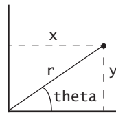
Polar coordinates
